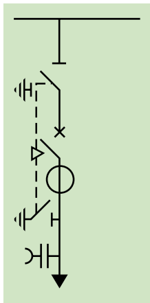
DM1-A Prekidačka jedinica
